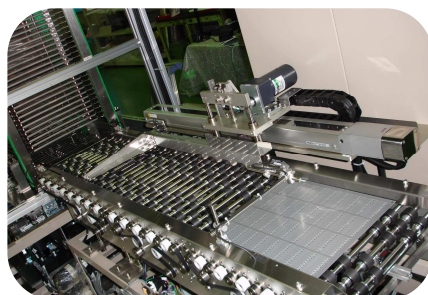
枚葉式縦型バッファー 搬送装置
